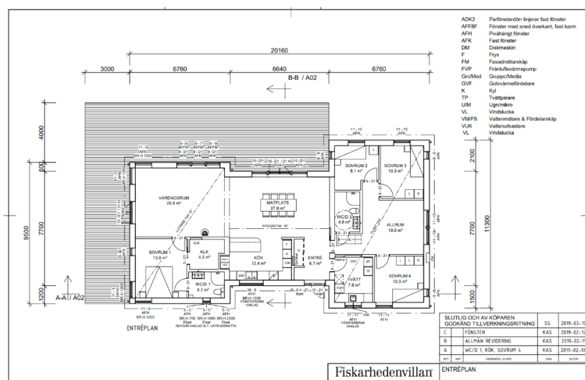
Figur 1: Planritning över testhus 1, Fiskarhedenvillans hustyp Brilljanten. Källa: Fiskarhedenvillan.
