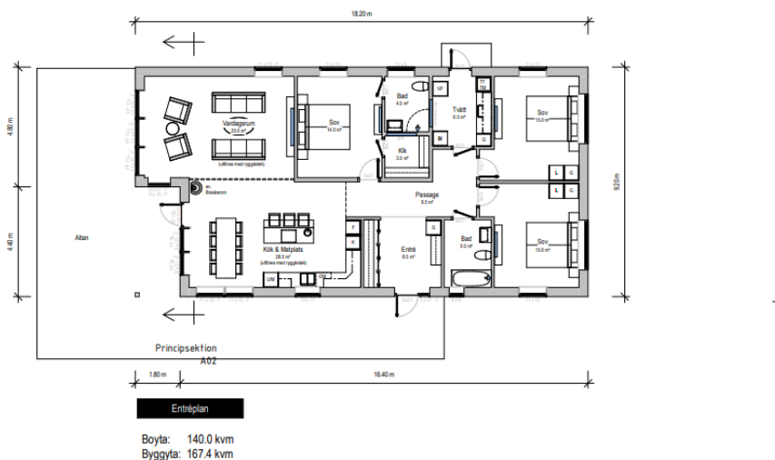
Figur 3: Planritning över testhus 2, Huspartners hus. Källa: Huspartner.
